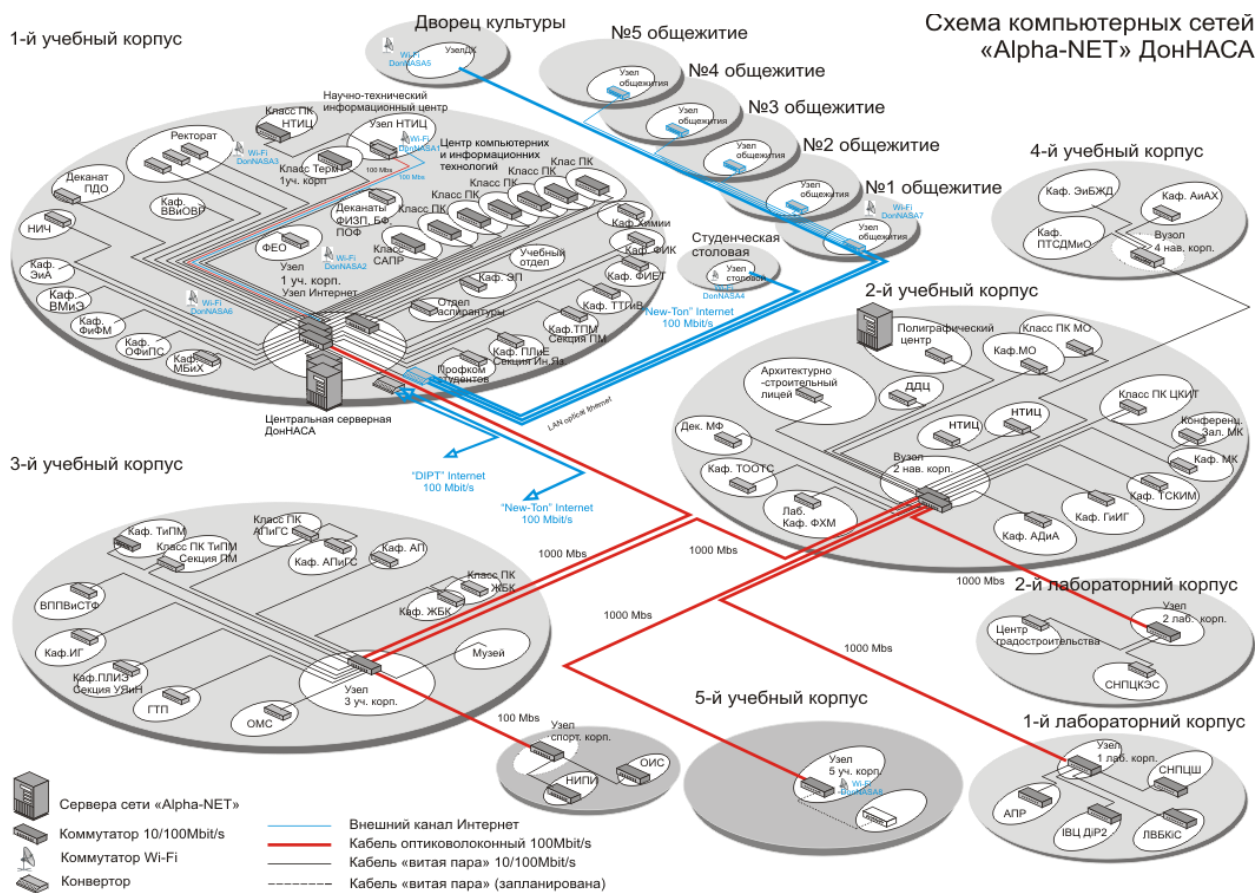
Рис. 6.5. Схема компьютерных сетей «Alpha-NET» ДонНАСА
