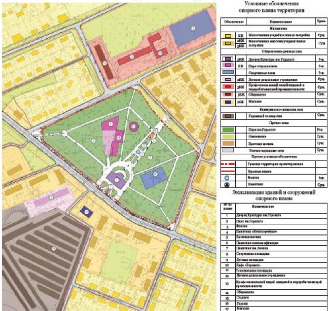
Рисунок 3. Схема опорного плана территории участка застройки
