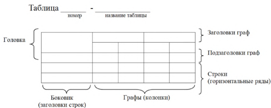
Рисунок 1 – Построение таблицы
