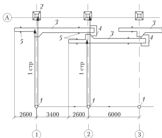
Рисунок 3.1 - Технологическая схема монтажа колонн способом «скольжения»:
